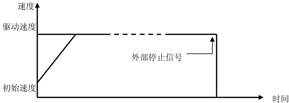
图 2.1.6 连续脉冲驱动
