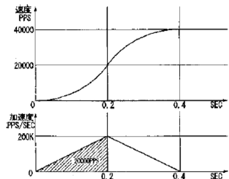
图 2.2.5 S 曲线加减速驱动
