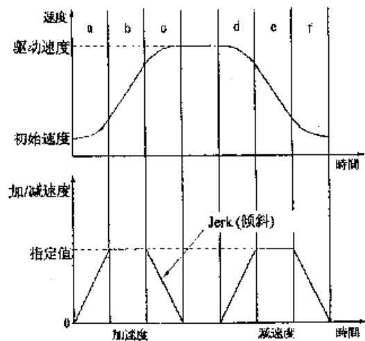
图 2.2.5 S 曲线加减速驱动
