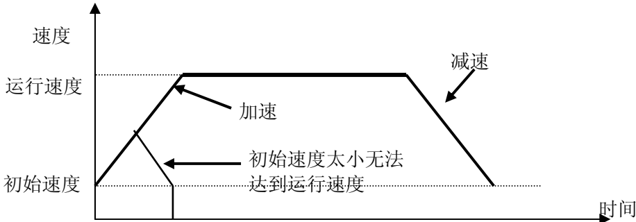
图 2.2.2 直线加/减速
