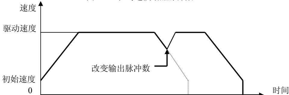
图 2.1.3 在降速段增加脉冲数
