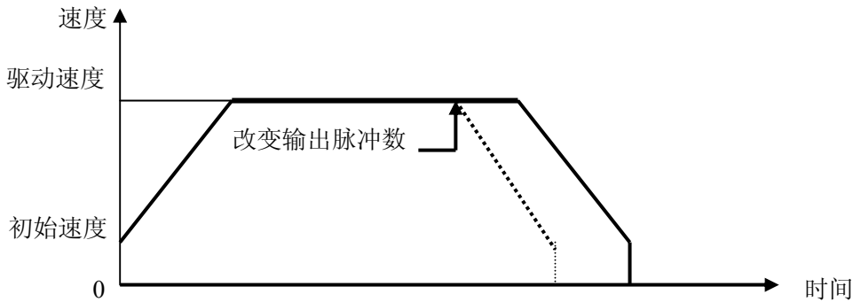
图 2.1.2 在匀速段增加脉冲数
