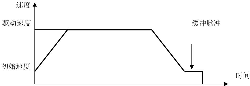
图 2.1.5 定长方式下的缓冲脉冲
